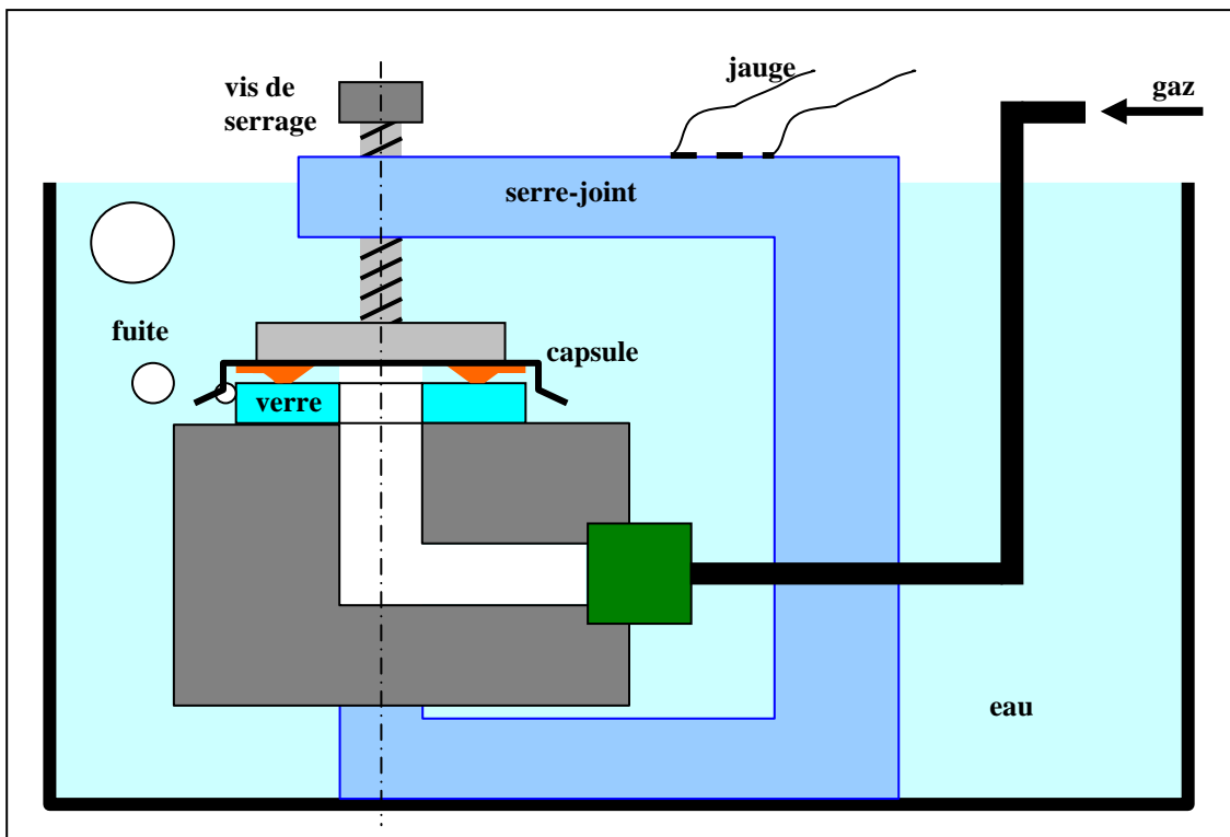
Figure 2.7 Test de fuite sur une surface plane Tirée de Champliaud (2000, p. 139)
